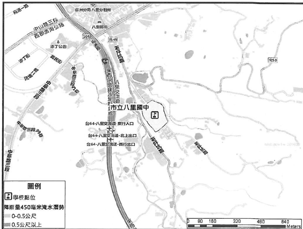
圖2.4.2 淹水災害潛勢圖 (瀏覽日期：109 年 9 月18 日)
