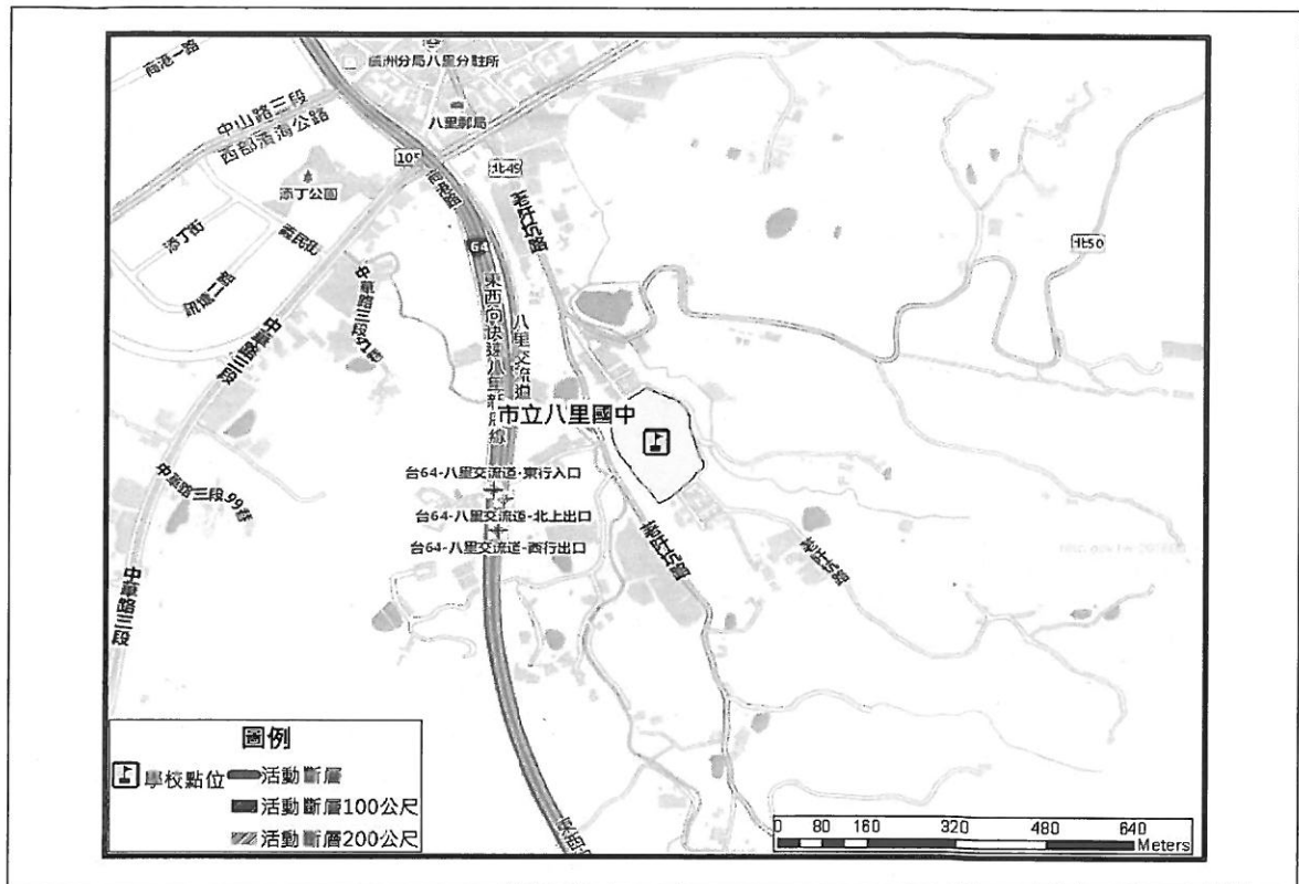
圖 2.4.1 地震災害潛勢圖 (瀏覽日期：109 年 9 月 18 日)
